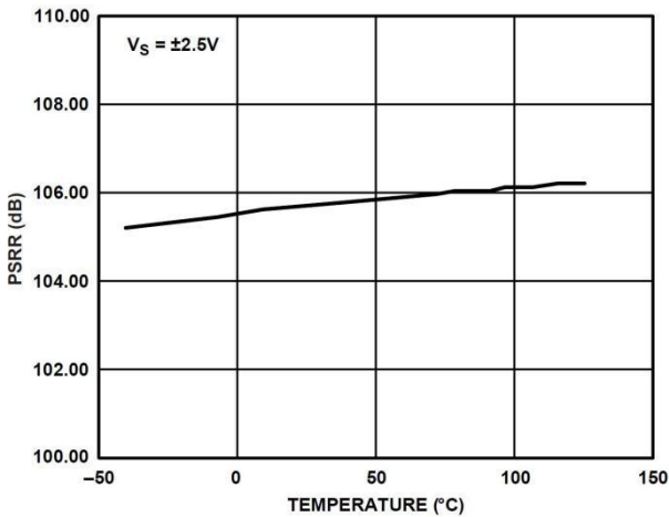
图 17.大信号 PSRR 与温度的关系
