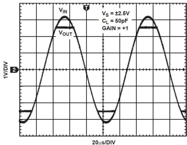
图 20. 无相位反转
