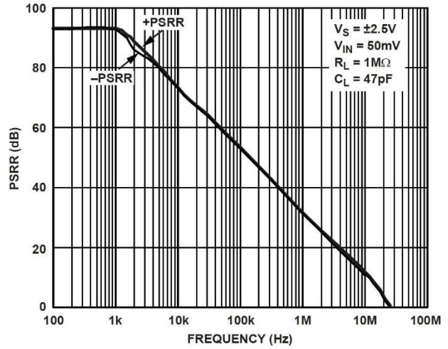
图 16. 小信号 PSRR 与频率的关系
