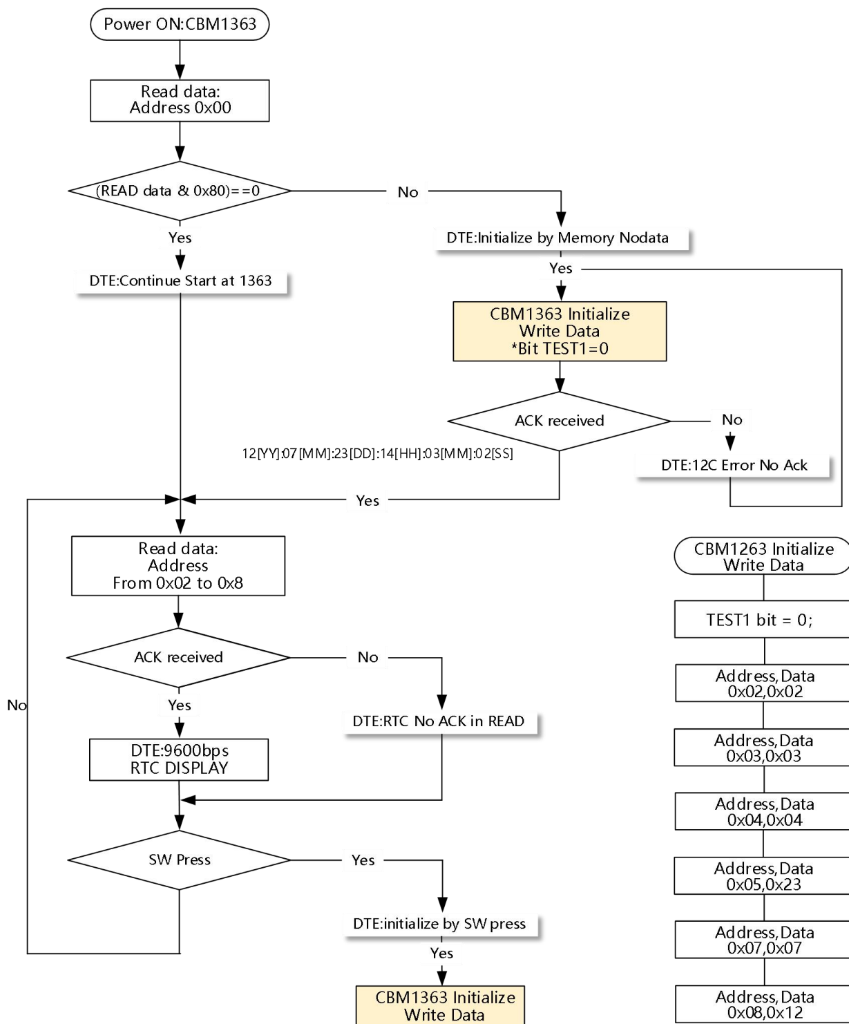
图 3. CBM1363 流程图
