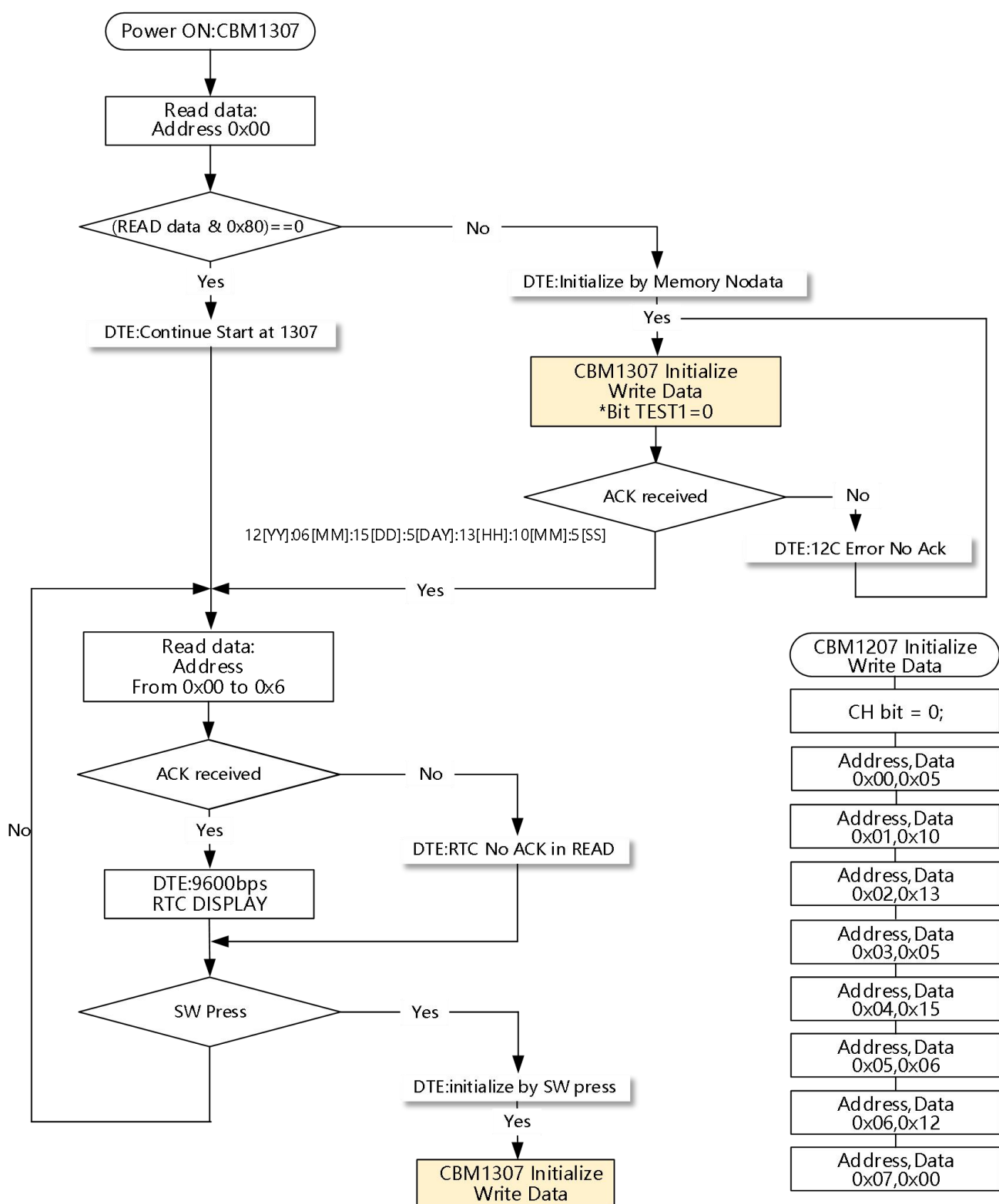
图 4. CBM1307 流程图
