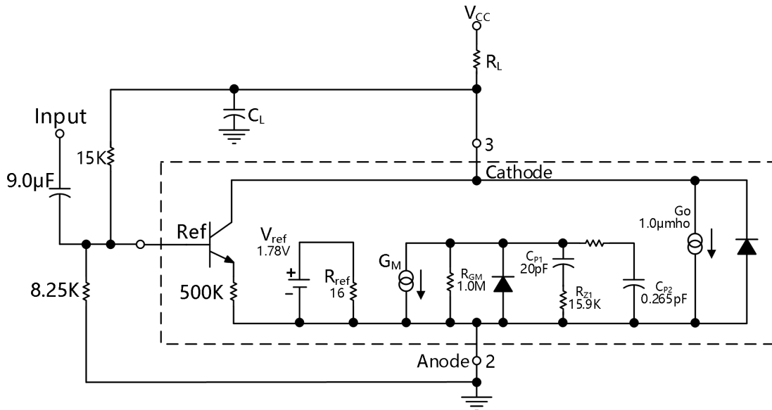
图 31.简化的 CBM432 设备模型
