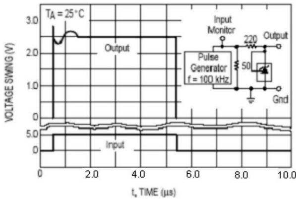
图 14. 脉冲响应
