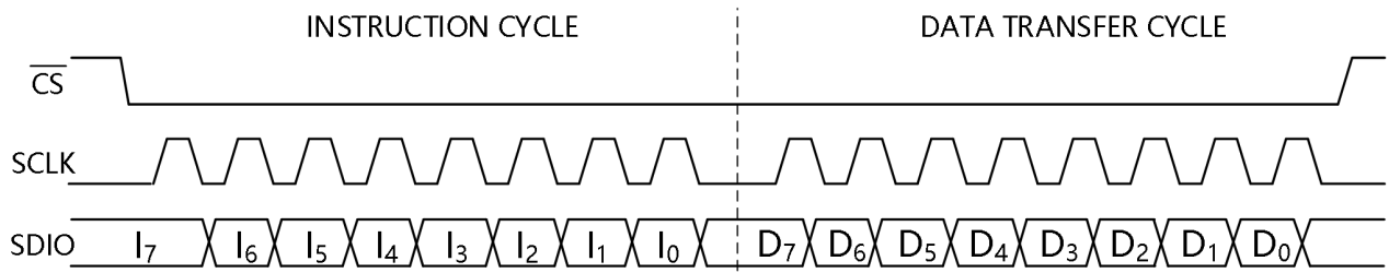
图 14 串行端口写入时序—时钟空闲为低
