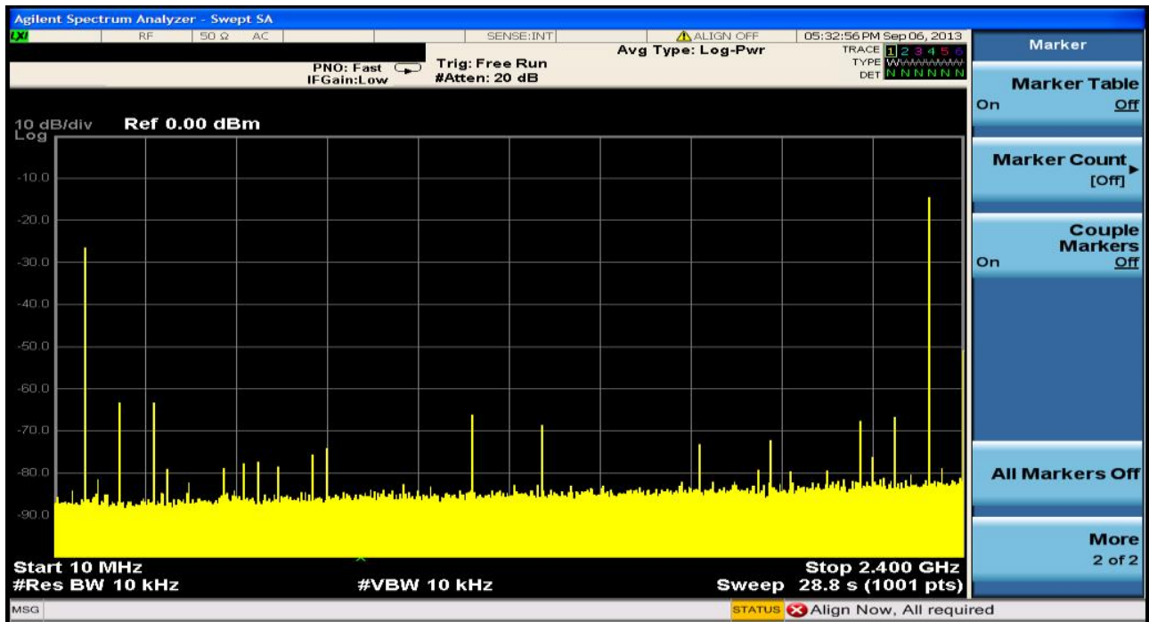
图 14 单音信号频谱, f_{\text{OUT}}=2.31\text{GHz} , f_{\text{DAC}}=2.4\text{GSPS}
