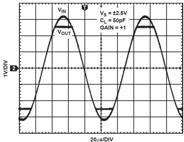
图 20. 无相位反转
