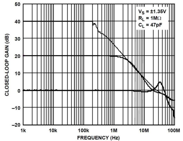
图 50. 闭环增益与频率的关系
