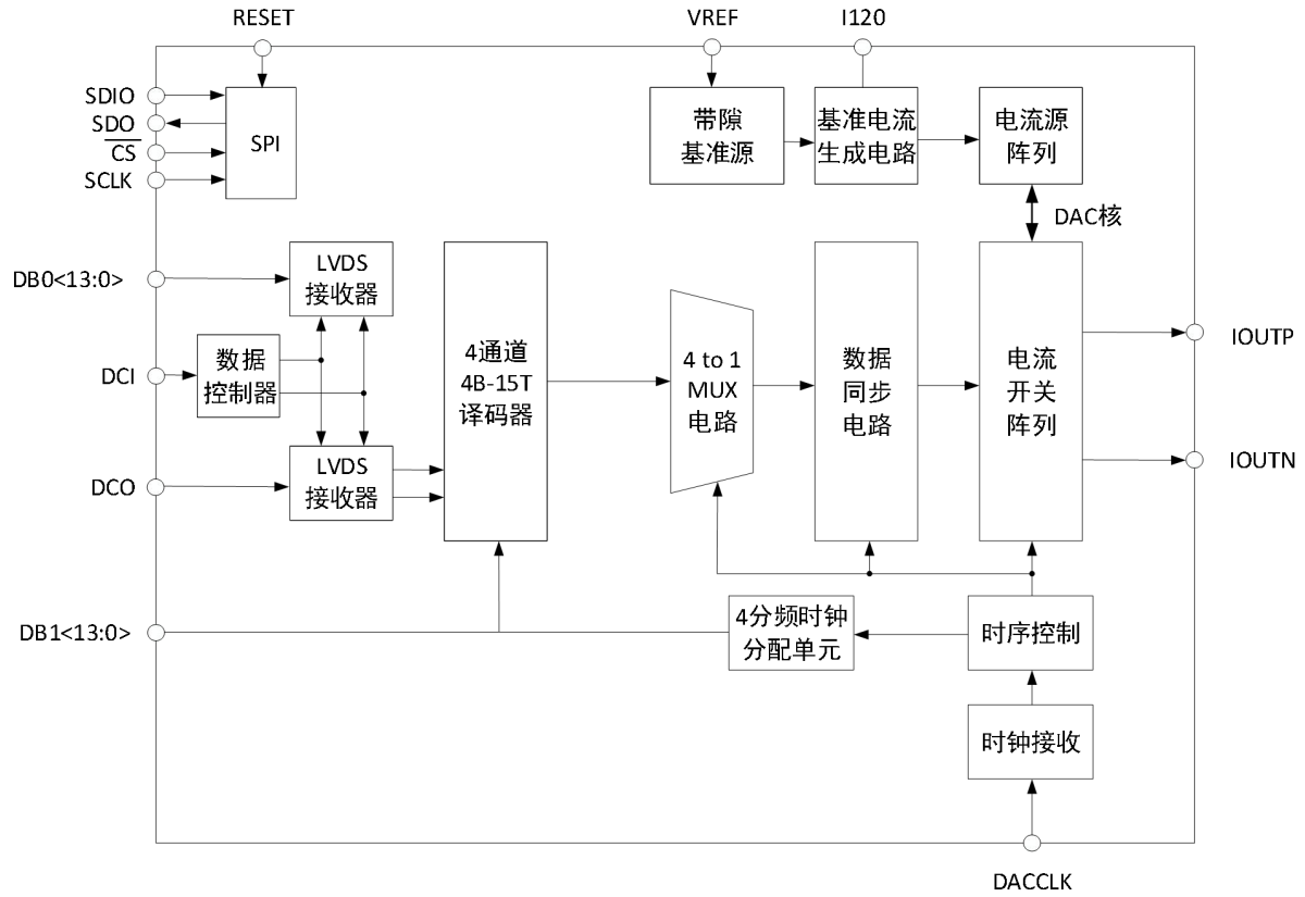
图 1. CBM97D39 功能框图
