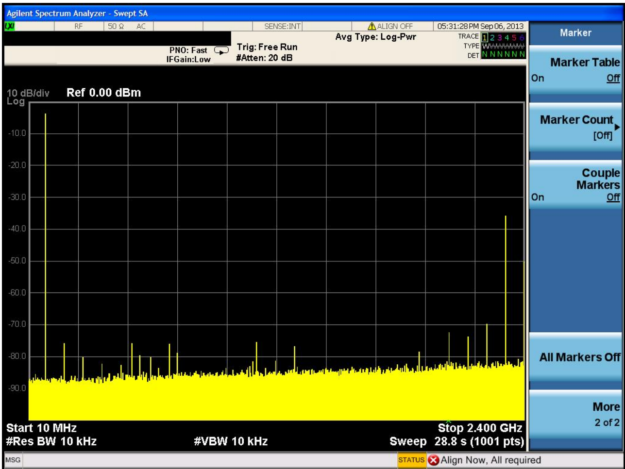
图 3 单音信号频谱, f_{OUT}=91\text{MHz} , f_{DAC}=2.4\text{GSPS}
