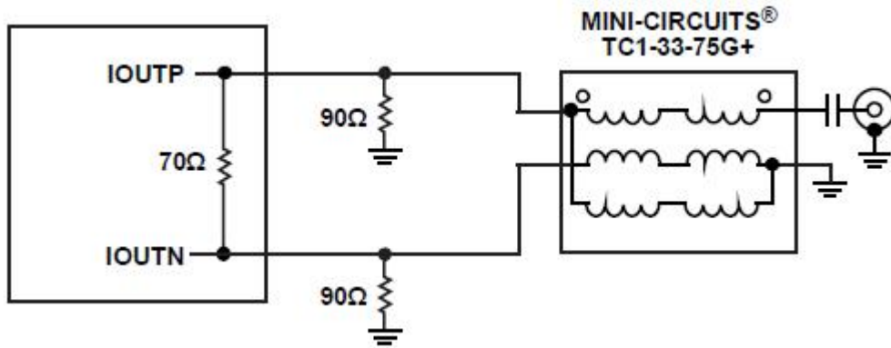
图 44 高达 2.2GHz 输出的推荐电路
