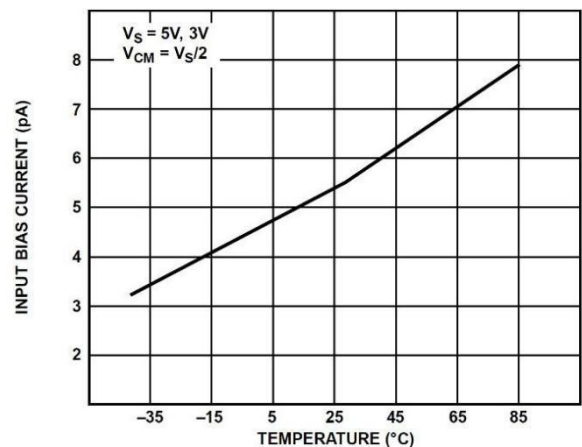
图 8. 输入偏置电流和温度的关系
