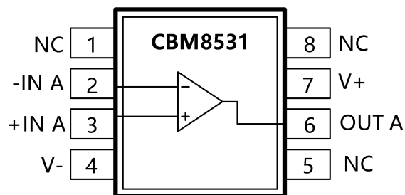
图 2 .SOP-8
