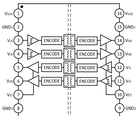
图 4. CBMuD1402
