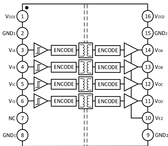
图 2. CBMuD1400
