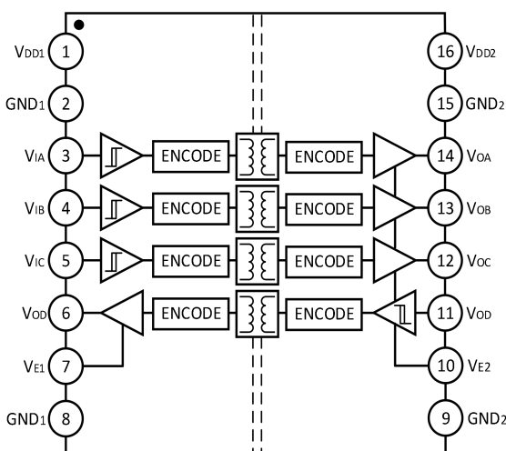
图 3. CBMuD1401
