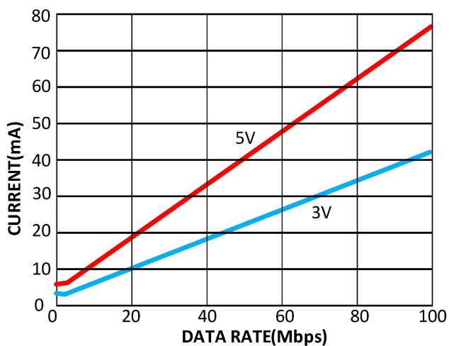
图 8. 典型的 CBMuD1400 V DD1 电源电流与数据速率的关系
