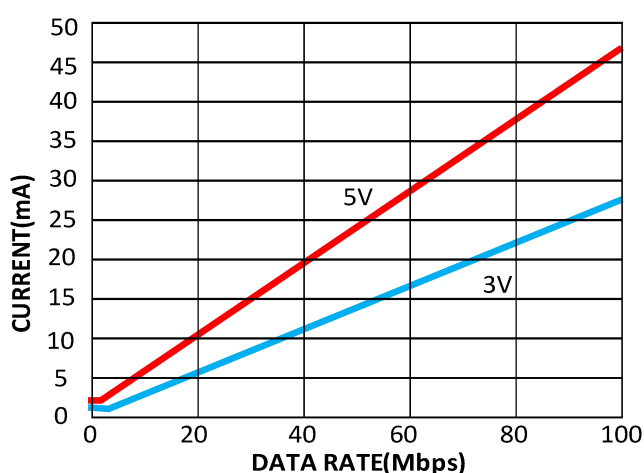
图 12. 典型 CBMuD1402 V_{DD1} 或 V_{DD2} 电源电流 与数据速率的关系
