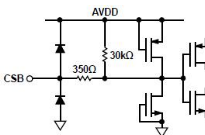
图 13. 等效 CS 输入电路
