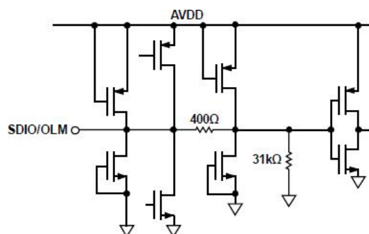
图 10. 等效 SDIO/OLM 输入电路
