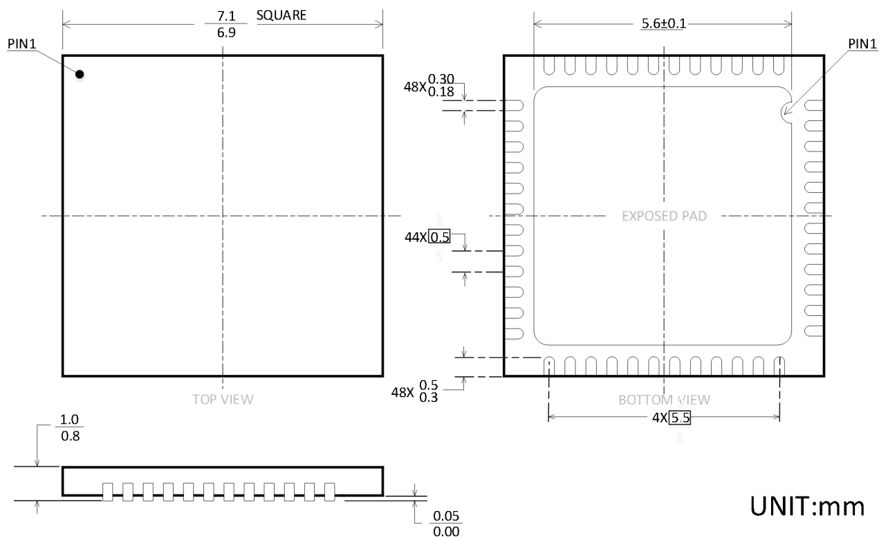
图 17. QFN-48 封装尺寸图
