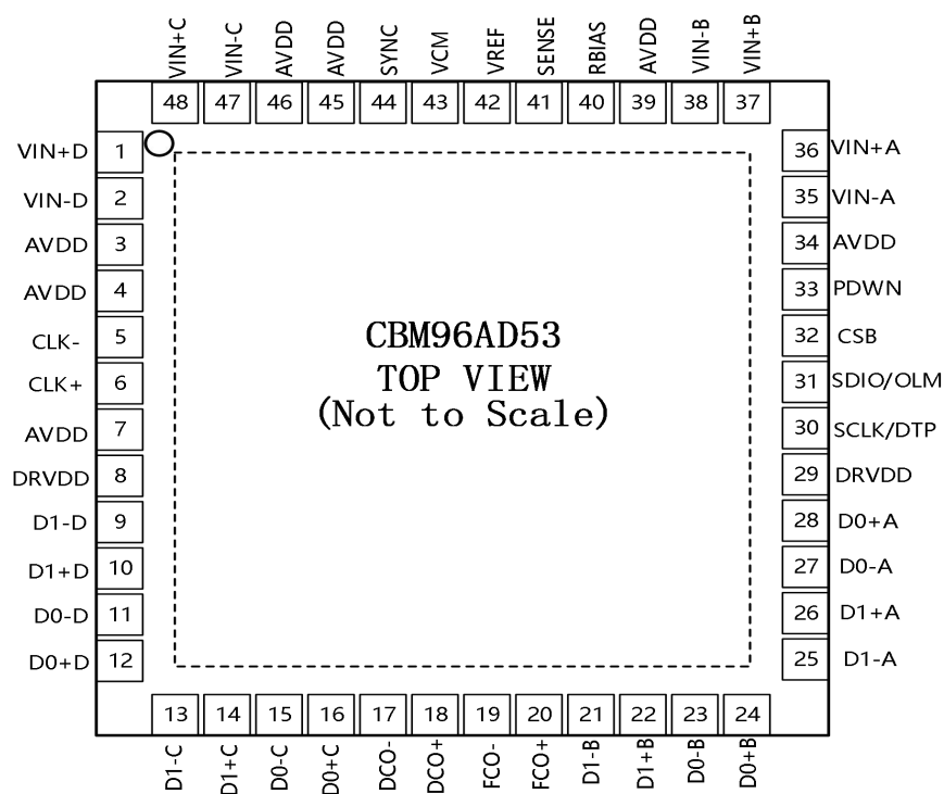
图 1. 引脚配置图
