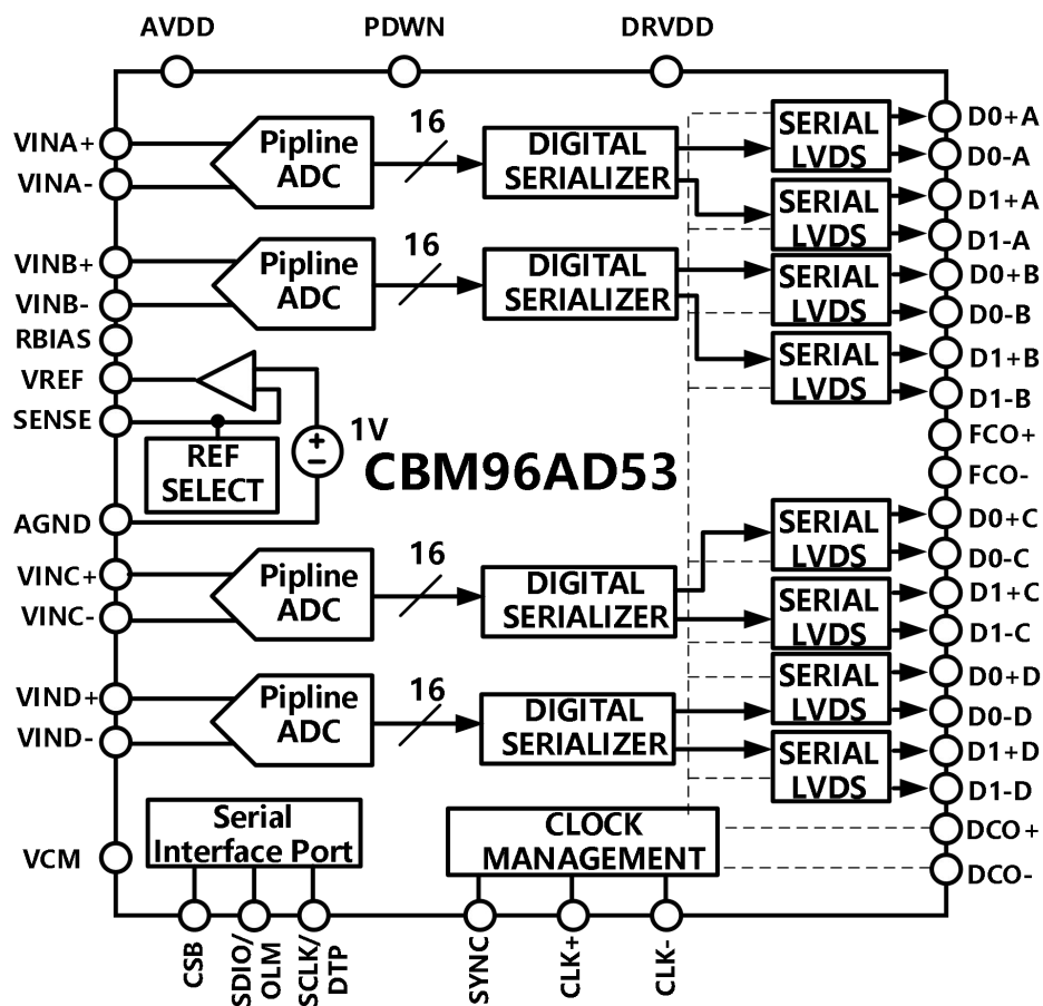
图 2. 功能框图
