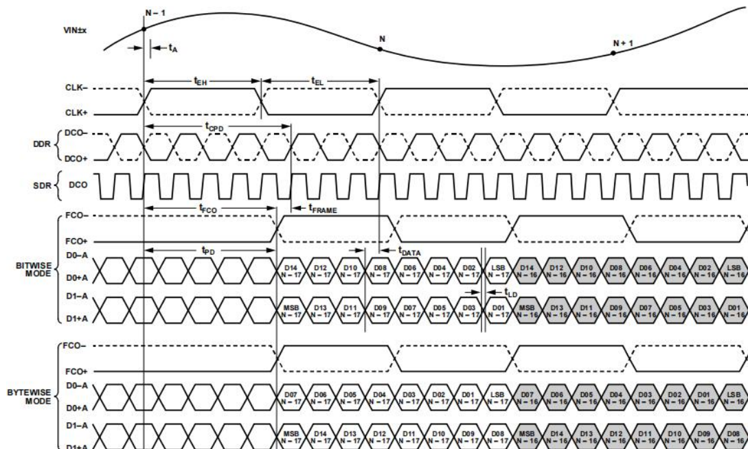
图 3. 16 位 DDR/SDR, 双通道, 1×帧模式 (默认)
