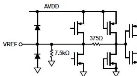
图 14. 等效 VREF 电路
