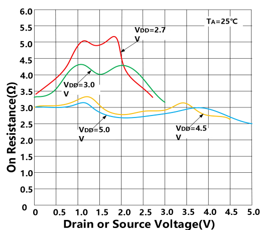
图 4.单电源下的导通电阻与 V_D ( V_S ) 的关系
