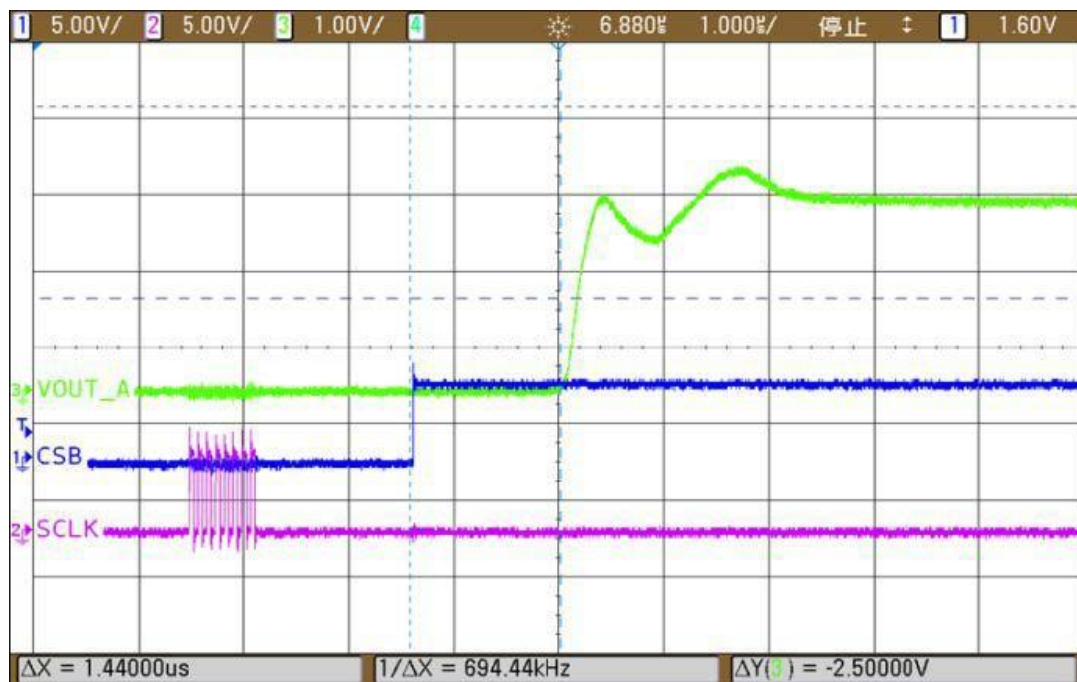
图 8. DAC 唤醒 (退出休眠状态) 过程
