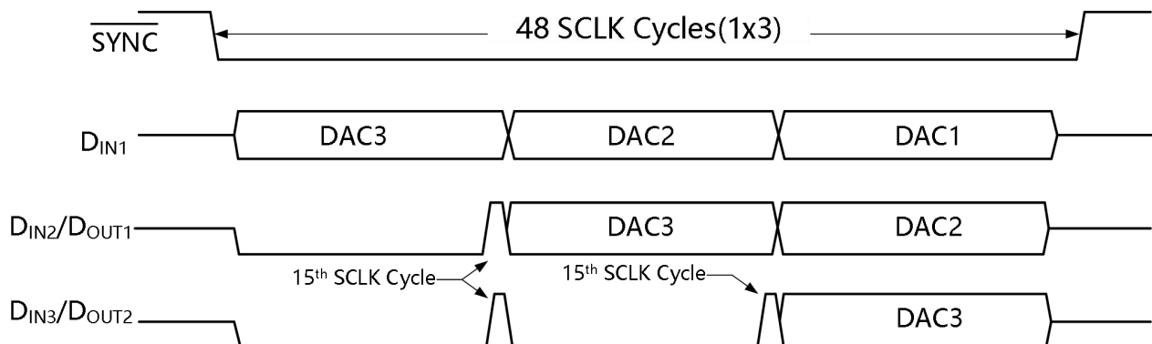
图 15.菊花链时序
