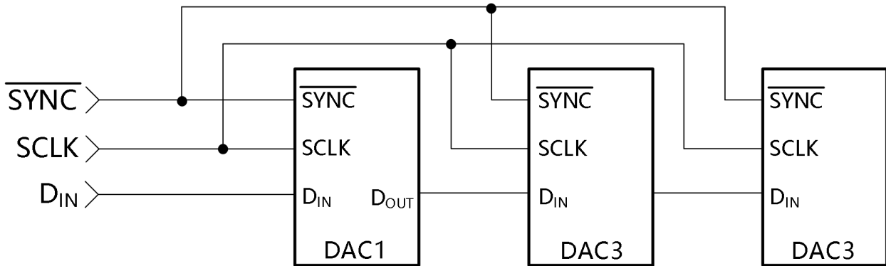
图 14.菊花链连接
