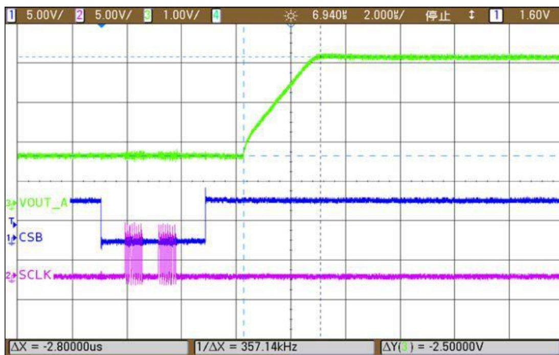
图 9. 输出建立过程 (0.25 满幅至 0.75 满幅变化)
