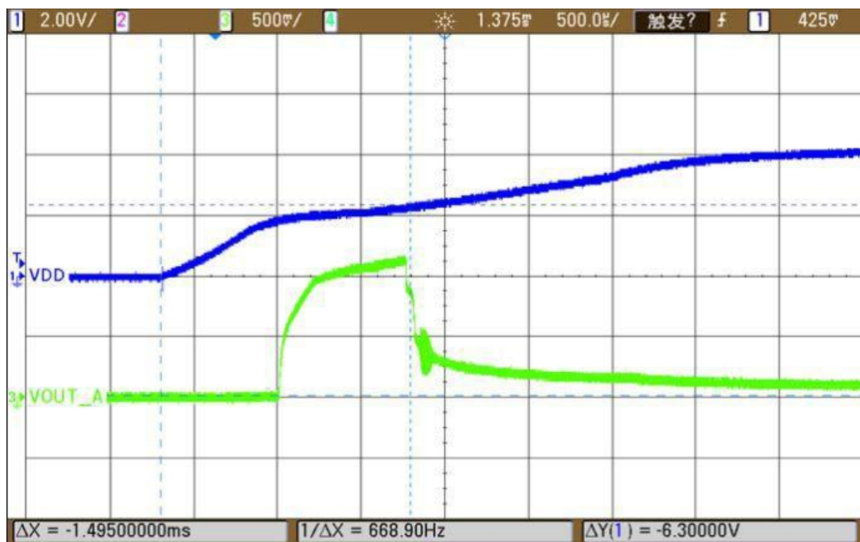
图 10. 上电复位
