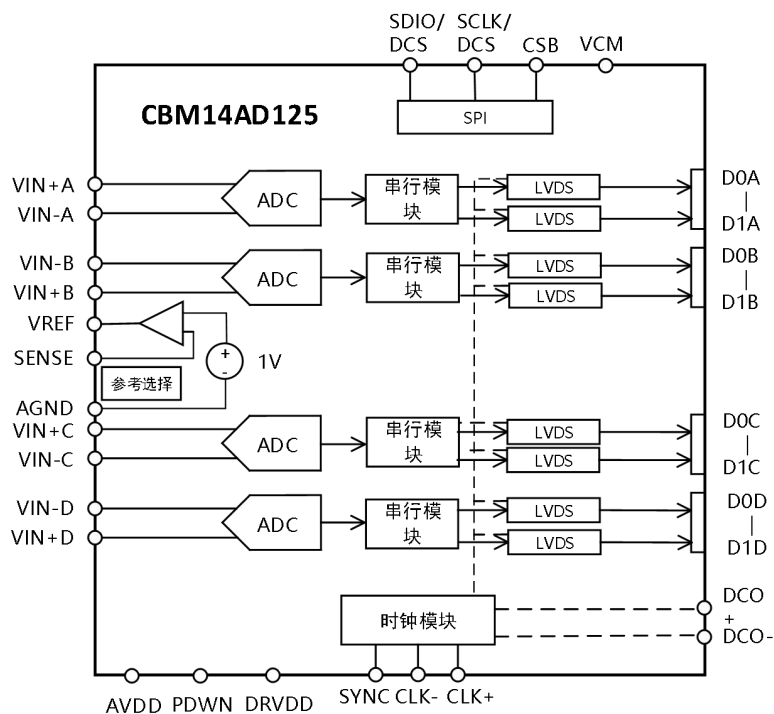
图 1. 功能框图
