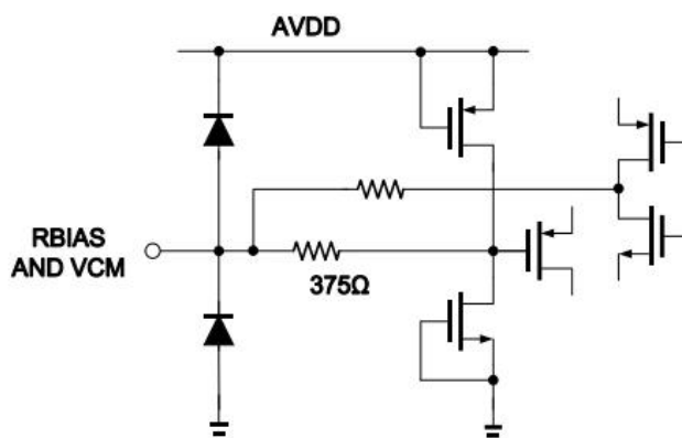
图 17 等效 RBIAS,VCM 电路
