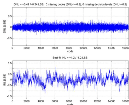
图 10. DNL/INL( f_{IN}=10MHz , f_s=125MSPS )
