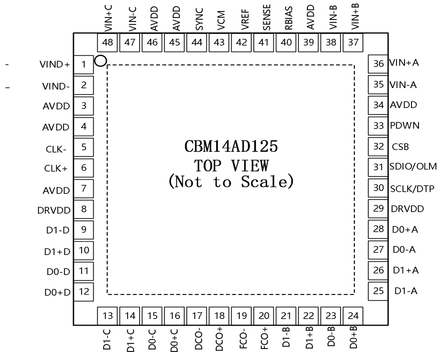
图 2. 引脚配置
