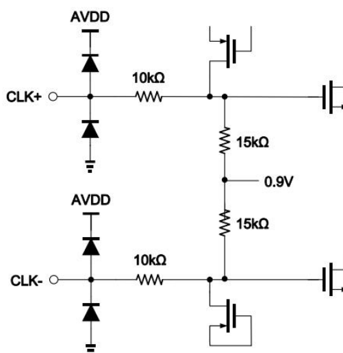
图 13 等效时钟输入电路
