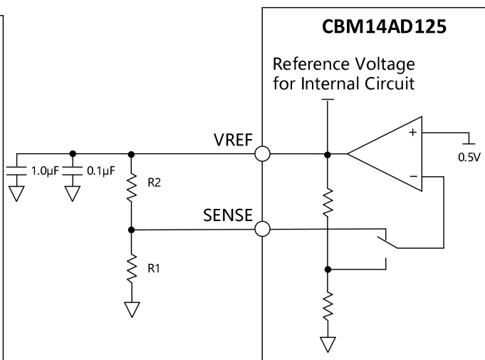
图 26. 外接电阻串模式 (VREF 外部配置模式)
