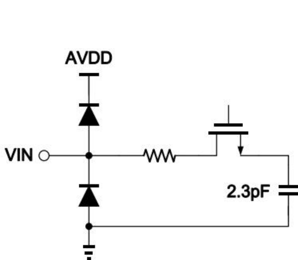
图 12 等效模拟输入电路
