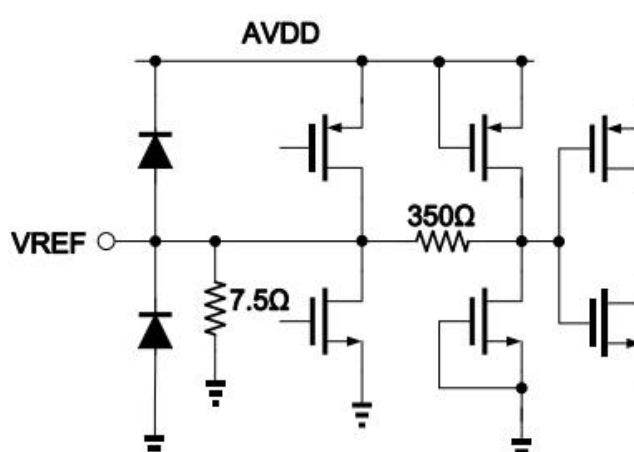
图 19 等效 VREF 电路
