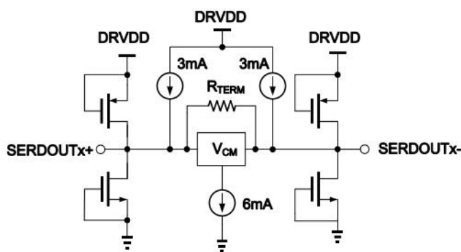
图 15 等效 SERDOUT±电路
