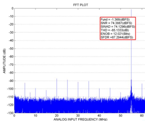
图 8. 单音 32K( f_{IN}=70MHz , f_s=125MSPS )
