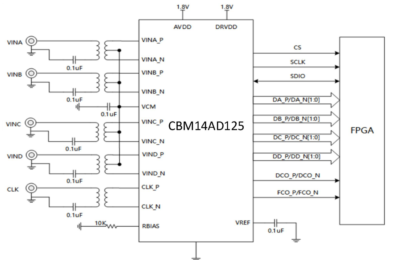
图 21 CBM14AD125 典型应用路线 (2Vpp 模式)
