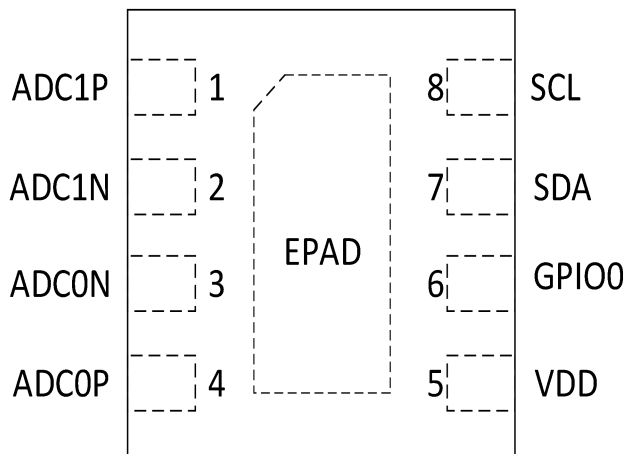
图 4 CBM12AD12D 引脚配置(A2) (俯视图)
