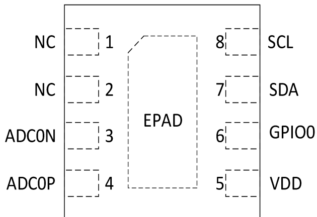
图 2 CBM12AD11D 引脚配置(A1) (俯视图)
