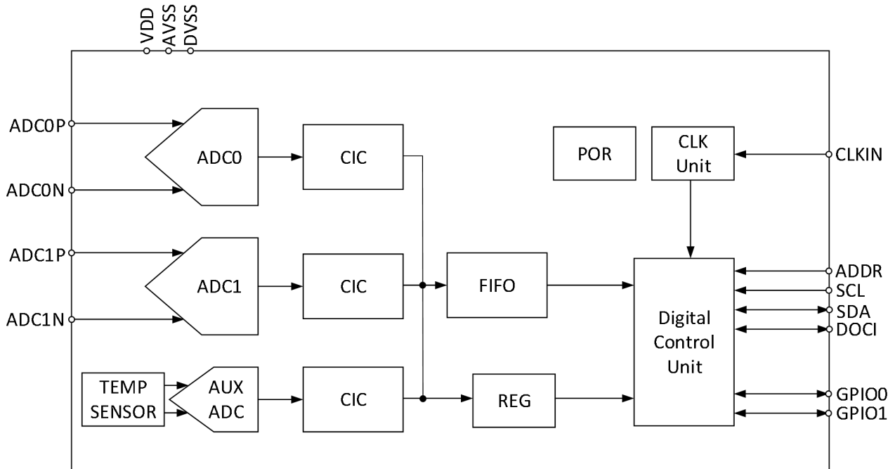
图 1 功能框图
