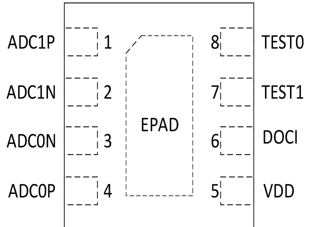
图 5 CBM12AD12B 引脚配置(B2) (俯视图)
