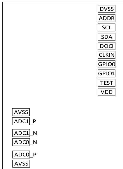
图 6 CBM12AD11/12-DIE 引脚配置(裸片) (俯视图)
