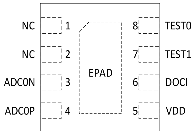
图 3 CBM12AD11B 引脚配置 (B1)(俯视图)
