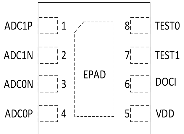
图 5 CBM12AD02B 引脚配置(B2) (俯视图)
