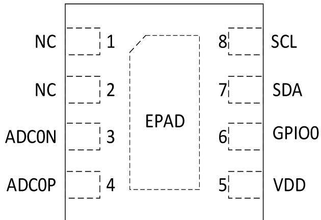
图 2 CBM12AD01D 引脚配置(A1) (俯视图)
