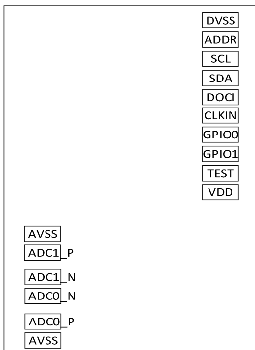
图 6 CBM12AD01/02-DIE 引脚配置(裸片) (俯视图)
