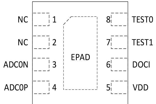
图 3 CBM12AD01B 引脚配置 (B1)(俯视图)
