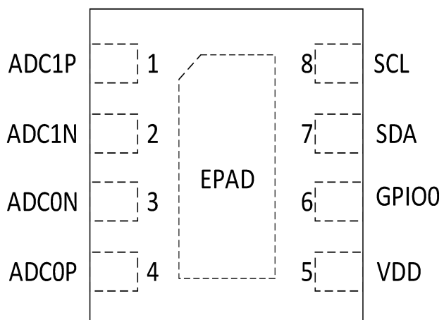
图 4 CBM12AD02D 引脚配置(A2) (俯视图)
