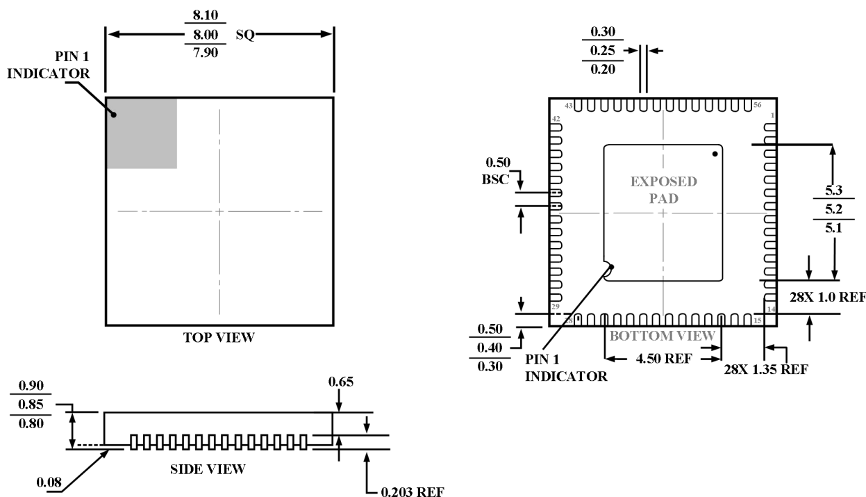
图 15. 外形尺寸图
