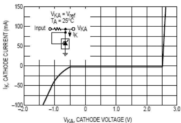
图 4. 阴极电流与阴极电压的关系
