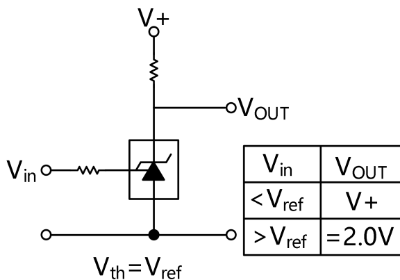
图 27. 温度补偿阈值单电源供电比较器
