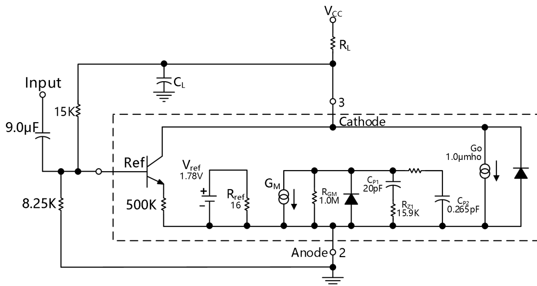
图 31.简化的 CBM431 设备模型
