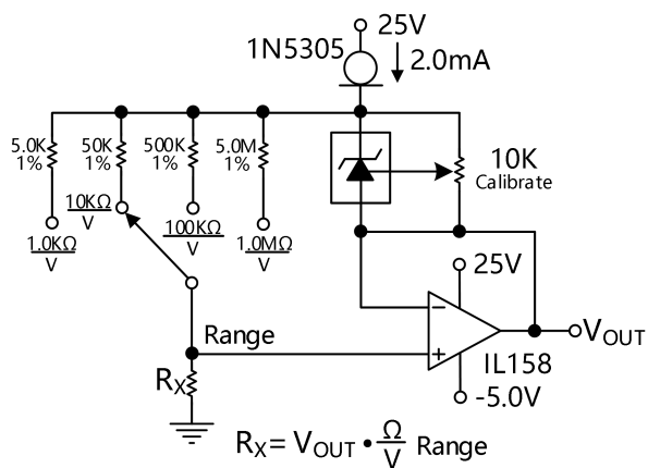
图 28. 线性欧姆计
