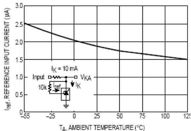
图 7. 基准输入电流与环境温度关系
