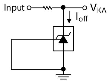
图 3. I_{off} 测试电路
