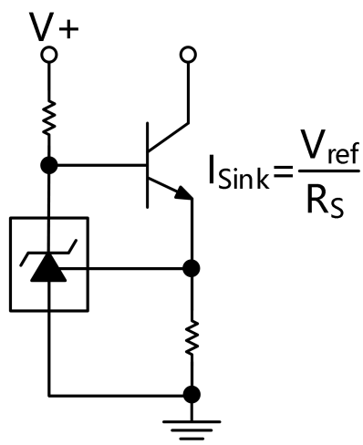
图 23. 恒定灌电流
