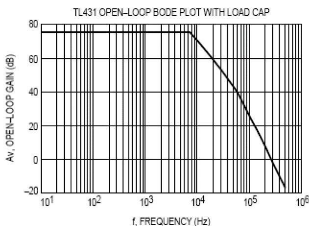
图 33. 例 2 开环增益电路
