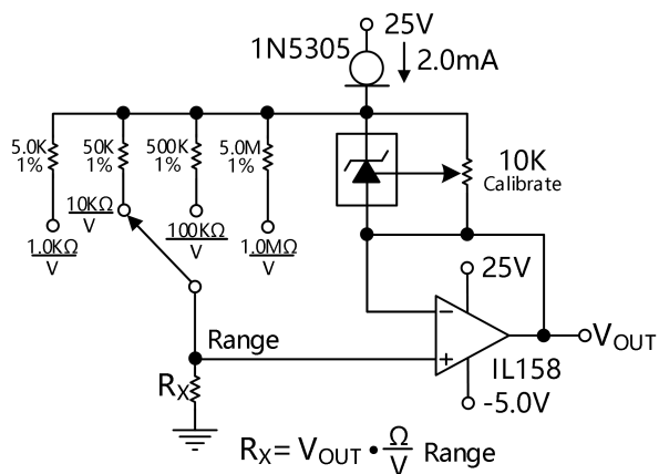
图 28. 线性欧姆计
