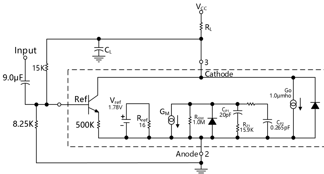
图 31.简化的 CBM432 设备模型
