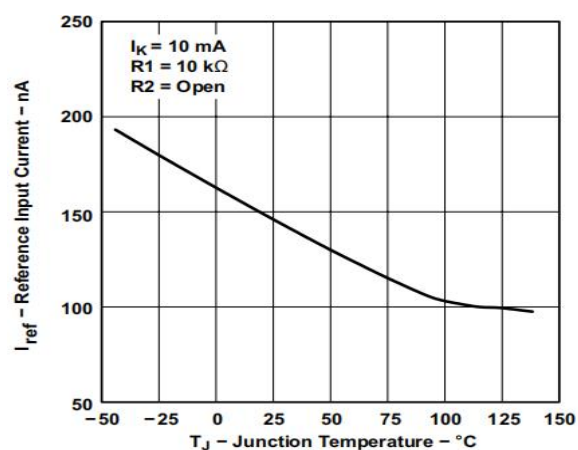
图 7. 基准输入电流与环境温度关系
