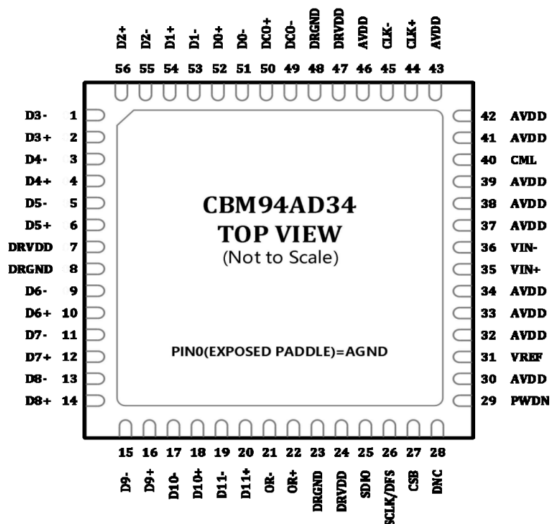
图 2.引脚配置图
