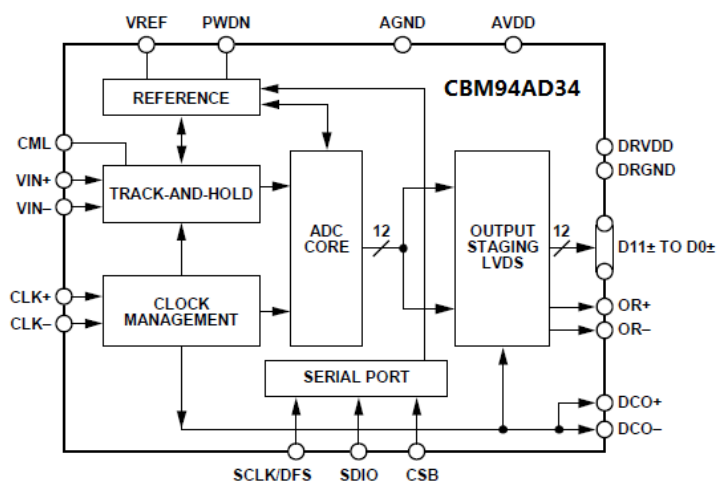
图 1.功能框图
