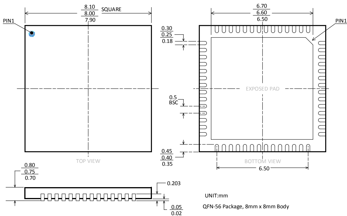
图 15. 外形尺寸图
